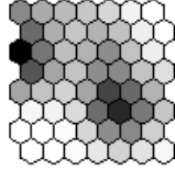
Lolium perenne
