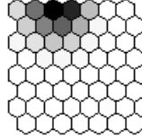
Festuca pratensis
