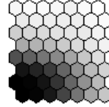
Festuca pseudovina
