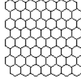
Hordeum jubatum
