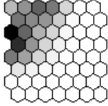
Poa angustifolia
