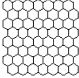
Eleocharis palustris
